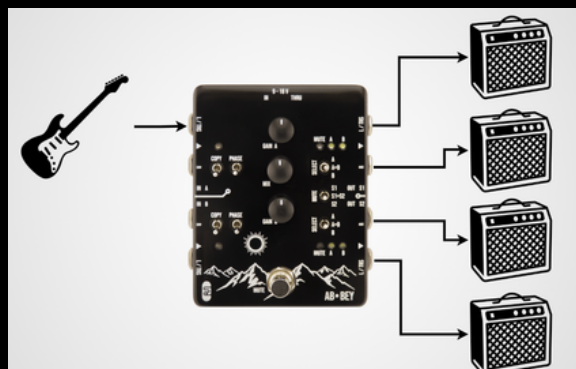
1 guitare sur 4 amplis
