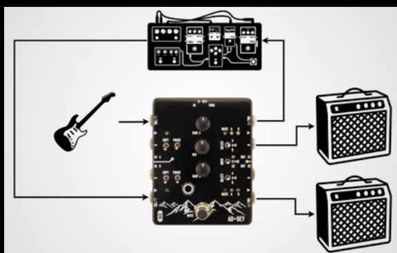
1 ampli DRY + 1 ampli WET / BLEND
